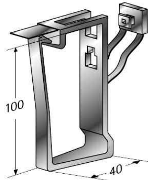
Kabelbügel - Kunststoff
